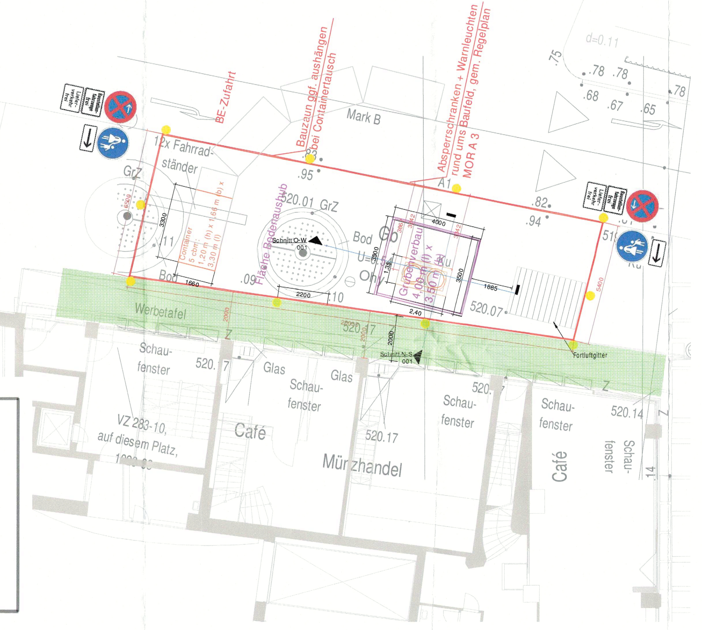
BE und Aufstellfläche Lüftungstürme M 1 : 100
