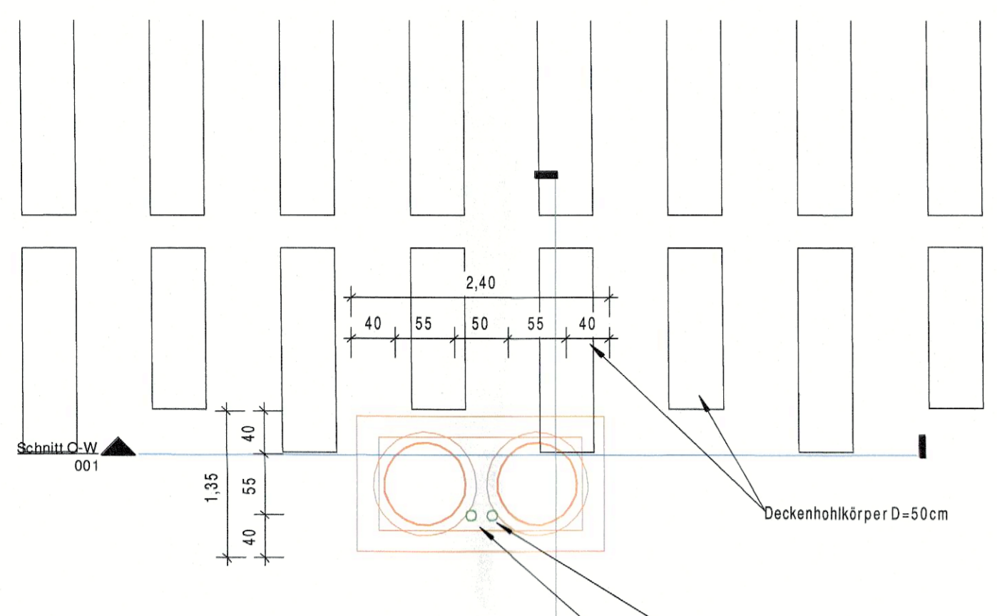
Grundriss M 1 : 50
