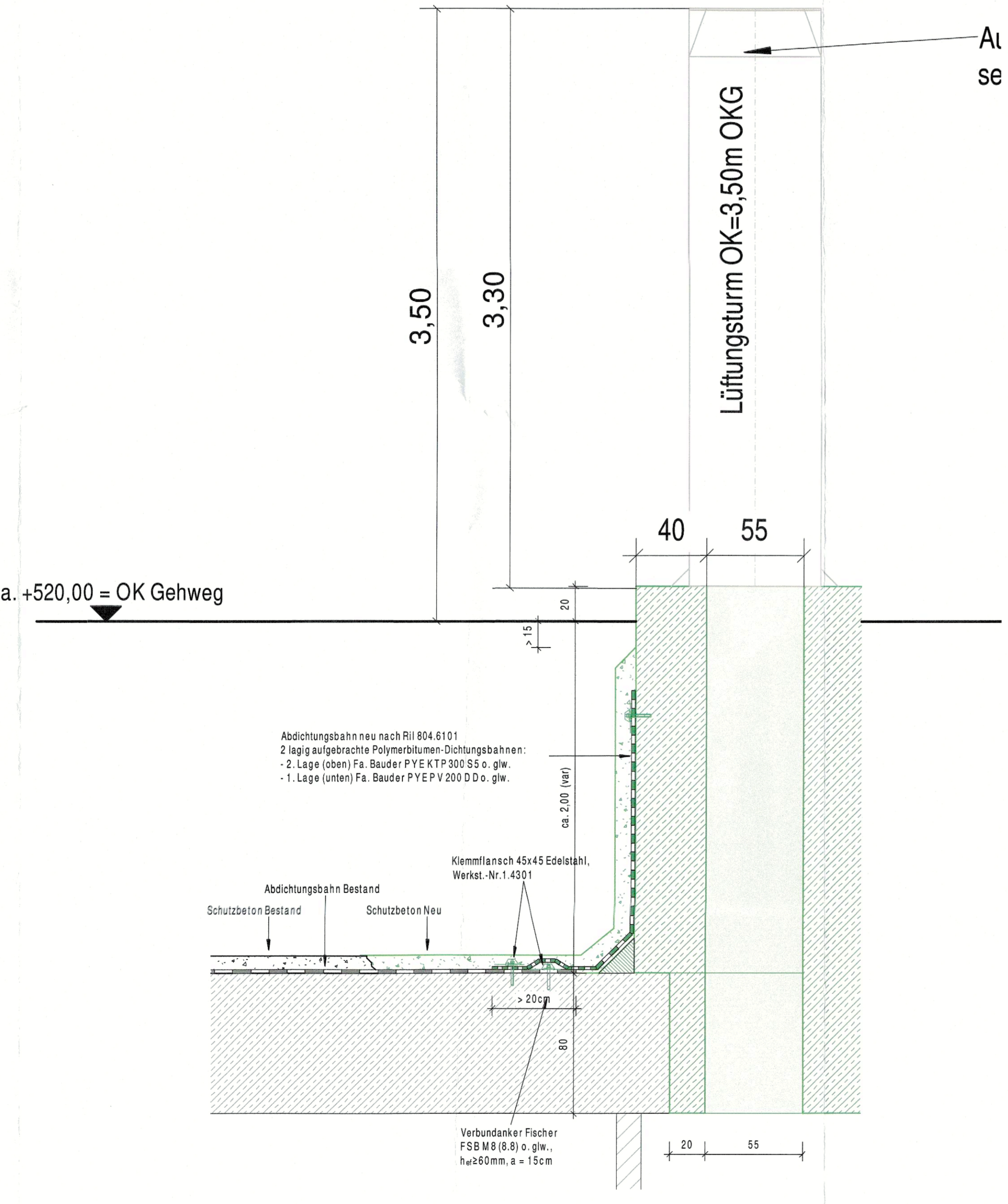
Detail Abdichtung M 1 : 20
