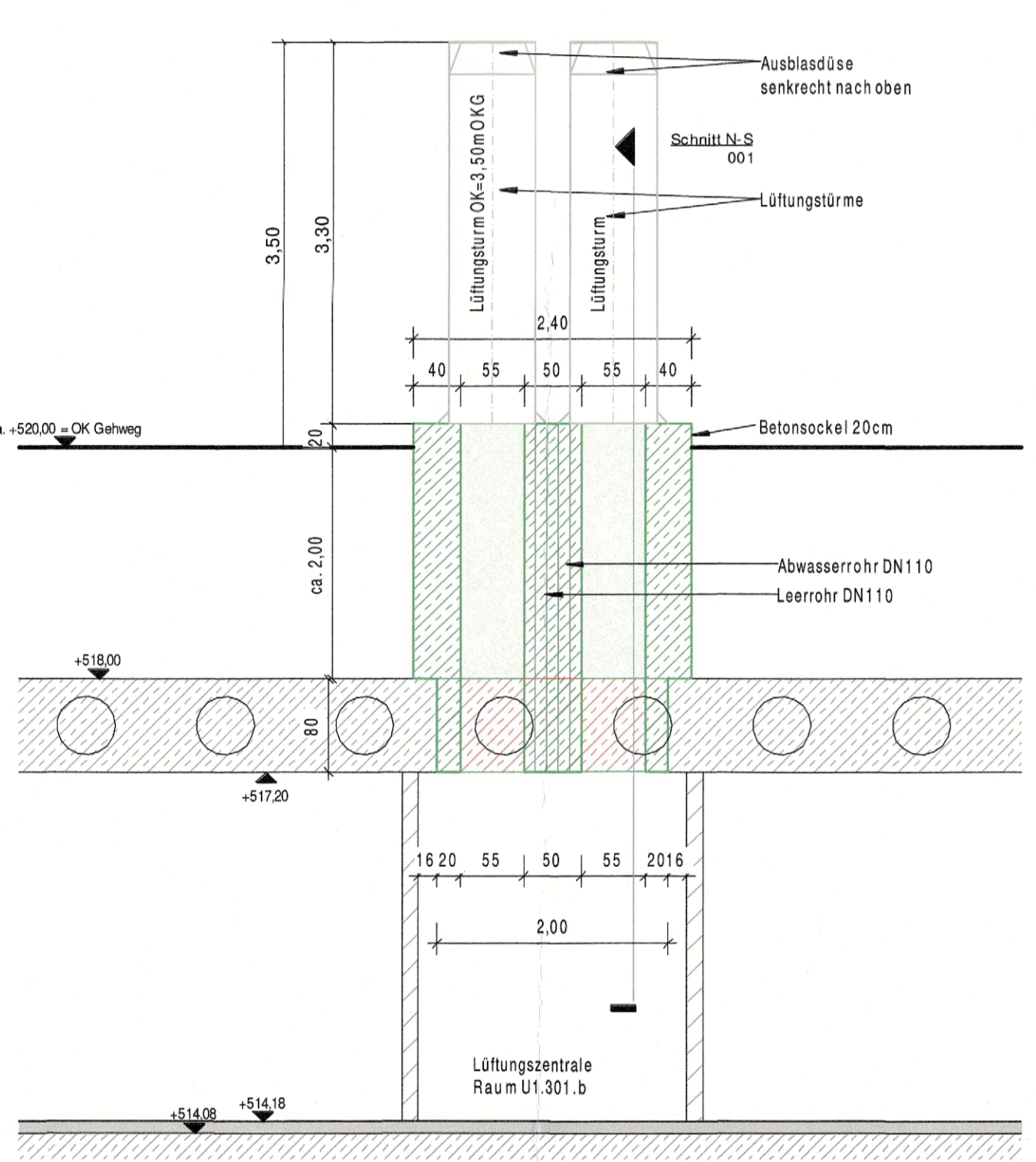
Schnitt O - W M 1 : 50
